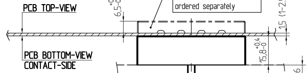
MiniSKiiP 2
