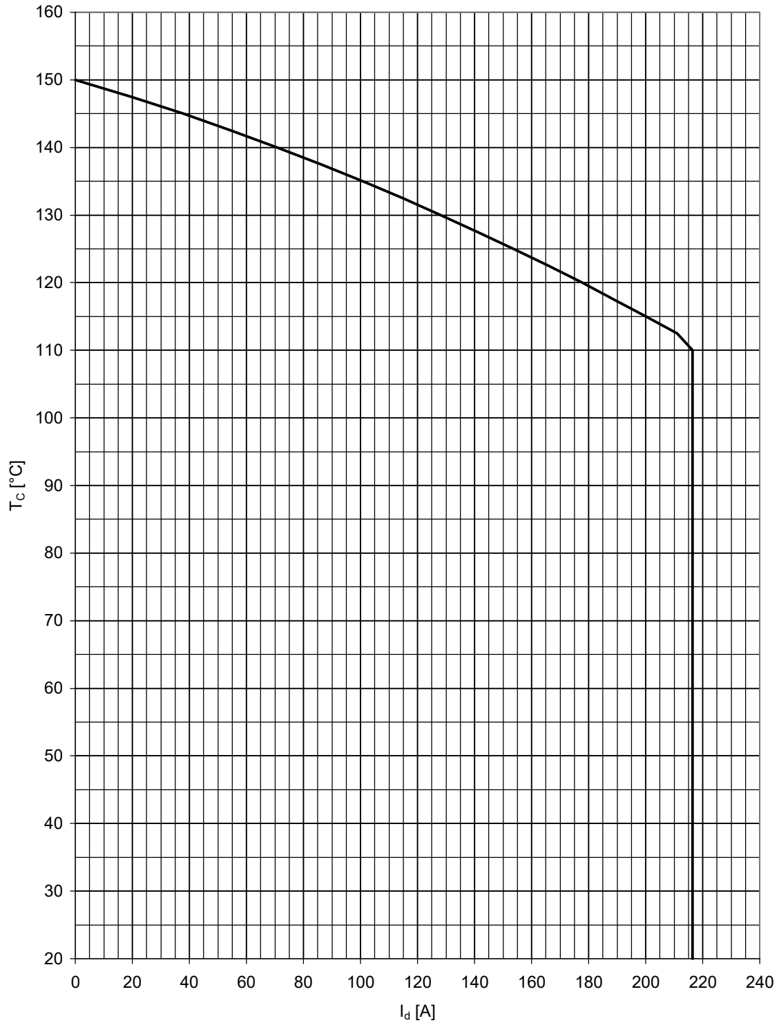
Höchstzulässige Gehäusetemperatur / Maximum allowable case temperature T_c = f(I_d)
